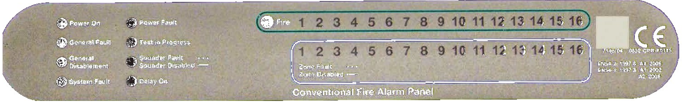
Şekil 1 — CF50016 ön panel gösterge ve kontrol arayüzü (16 zon)
